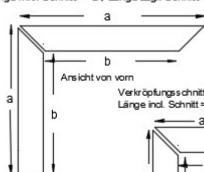
Gehrungsschnitt für Fensterumrahmung Länge inkl. Schnitt = a, Länge zzgl. Schnitt = b
