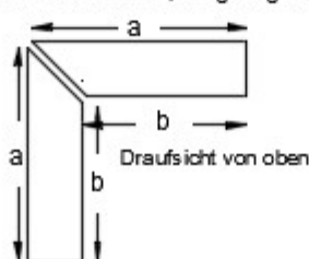
Verkröpfungsschnitt für Hausecken Länge inkl. Schnitt = a, Länge zzgl. Schnitt = b
